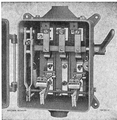
Coffret de manœuvre du type L, ouvert.
