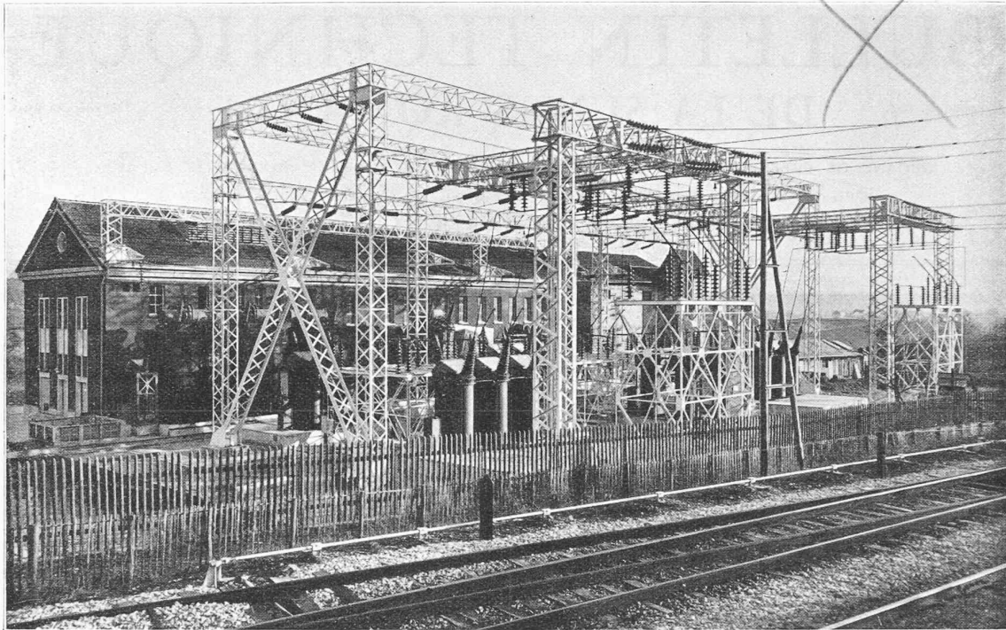
Fig. 15. — Vue du poste à 120 000 volts.
