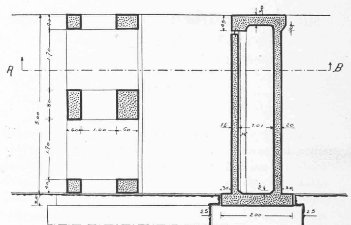
SEZIONE C - D
