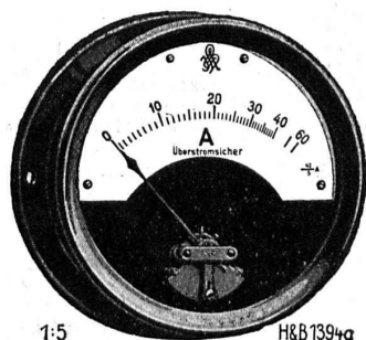
Ampèremètre de fer doux surchargeable "Fy".
