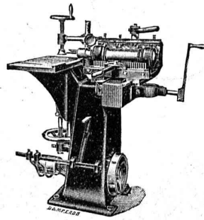
Mortaiseuse.
