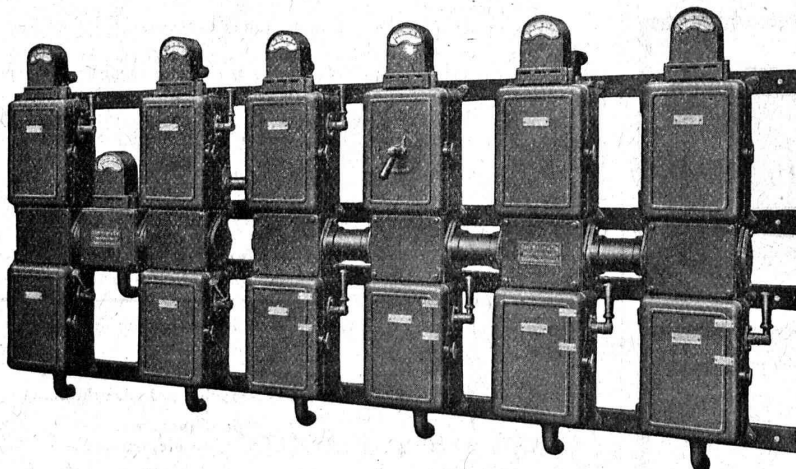
Batterie de coffrets de manœuvre.
