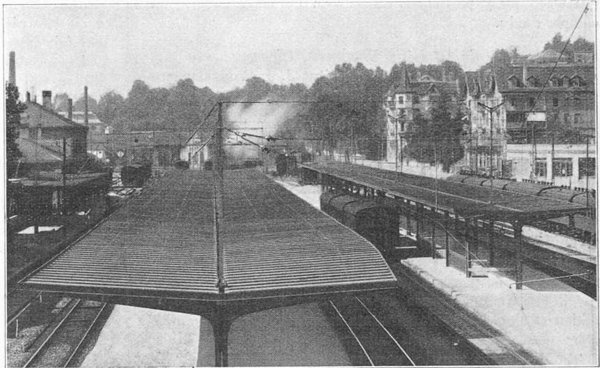
Fig. 4. — Marquises de la nouvelle gare de Fribourg, couvertes au moyen de plaques de cuivre « Debex ».
