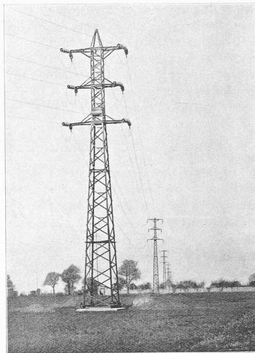
Fig. 4. — Ligne Peuffeyre-Malupalud-Montcherand. Pylône tenseur dans la plaine du Rhône.
