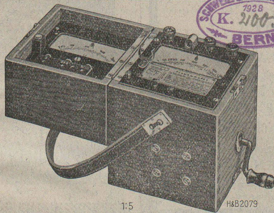
Mesureur d'isolement avec voltmètre.
