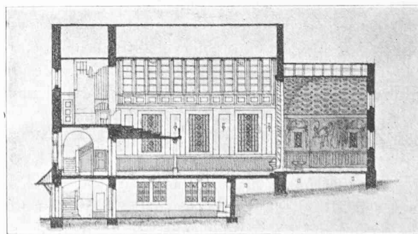
Coupe longitudinale. — 1 : 400.
