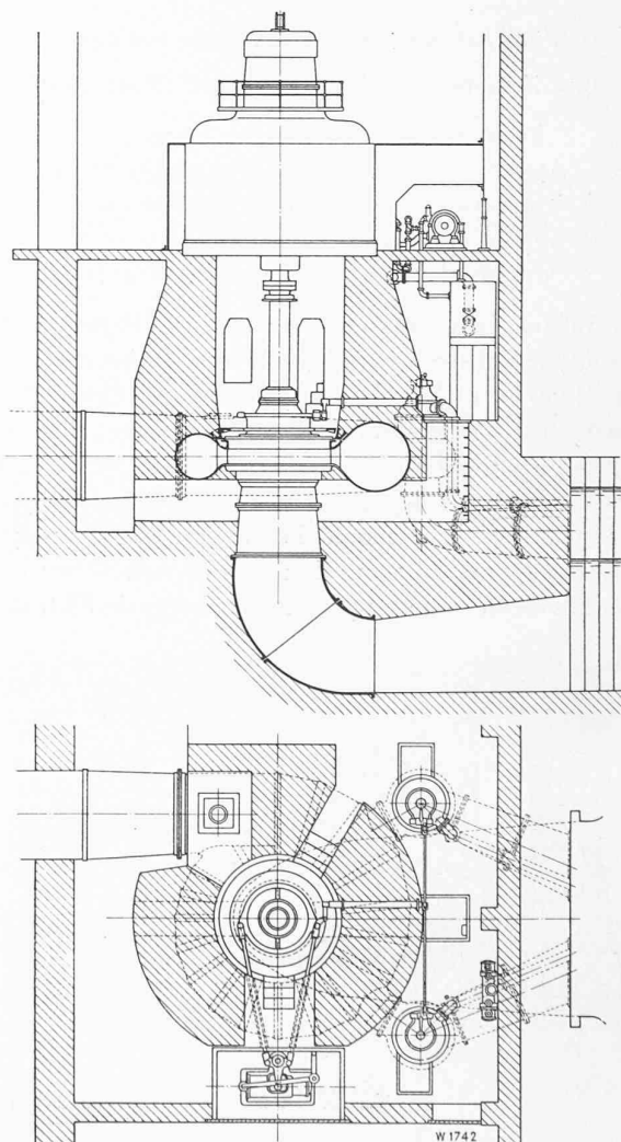
Fig. 5 et 6. — Turbine de Komaki (Escher, Wyss & Cie).
