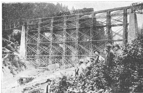
Fig. 35. — Viaduc de Czorbodom dans les Beskides, réparé par un pont provisoire de 5+7x10+5 m. Longueur totale 80 m.
