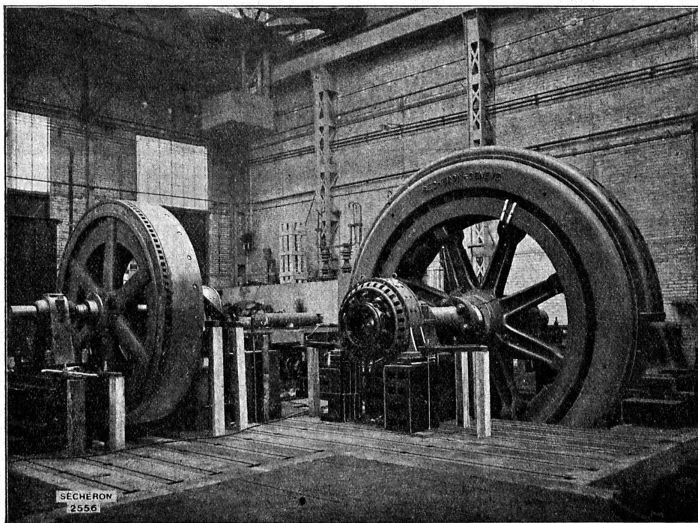
Ateliers de Sécheron. — Stand d'essai des machines tournantes.
