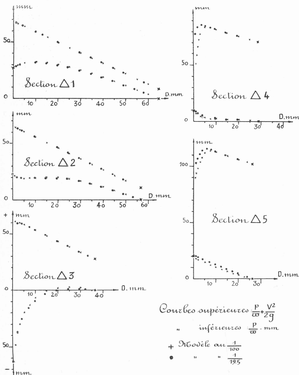
Fig. 14. — Répartition des pressions et de l'énergie aux divers points des sections Δ.
