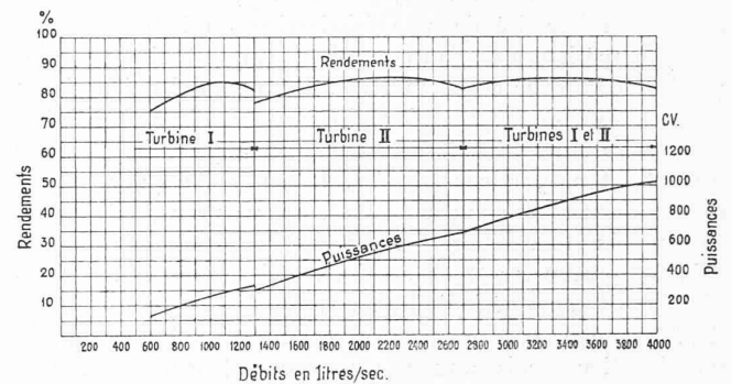
Fig. 1. — Centrale automatique de St-Sulpice. Rendements et puissances des deux turbines.
