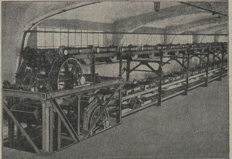
Chaîne à godets „Bleichert“ pour alimentation de chaudières (rendement 28 t à l'heure).
