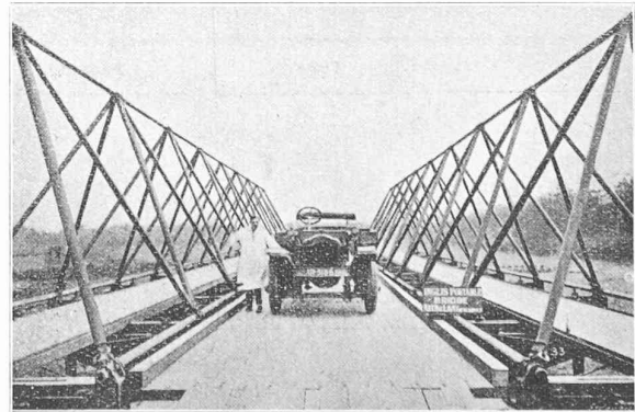
Fig. 21. — Pont système Inglis, composé de deux passerelles et d'un tablier intercalé.
