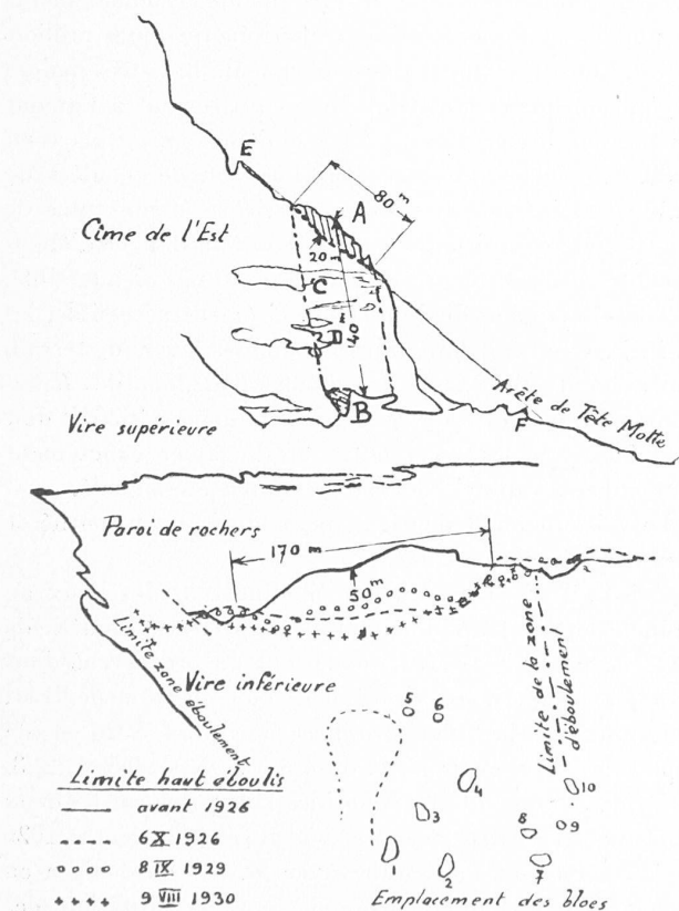
Fig. 3. — Région de formation des coulées du St-Barthélemy.
