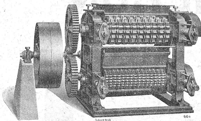
Concasseur à cylindres dentés.
