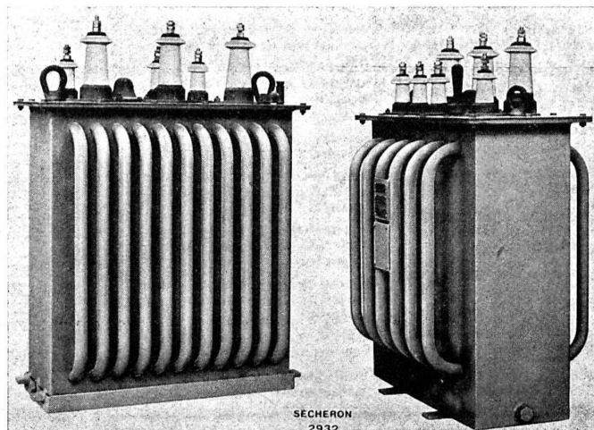
Transformateurs triphasés à cuve à tubes de refroidissement; à gauche, type pour montage à ciel ouvert, environ 75 kVA; à droite type pour montage sous toit, environ 30 et 50 kVA
