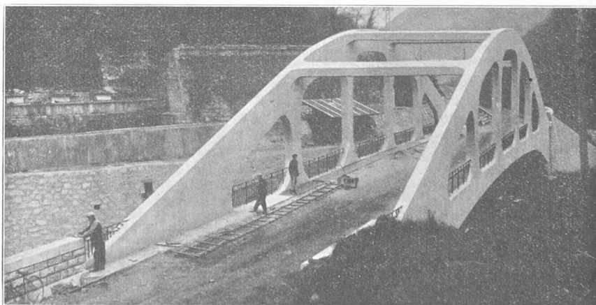
Fig. 10. — Pont de Naou-Hounts. Un aspect du pont terminé.
