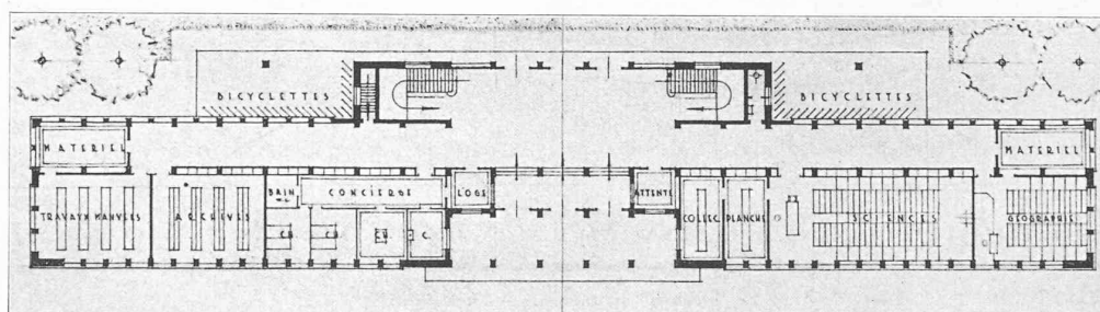
Plan du rez-de-chaussée. — 1 : 600.
