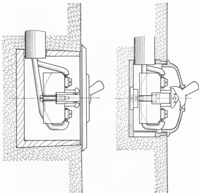
Fig. 5. — Montage encastré. Hauteur de la boîte 45 mm et 38 mm. Fig. 6. — Montage semi-encastré. Hauteur de la boîte 30 mm.
