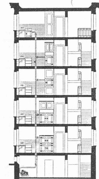
Fig. 1. — Installation « Froid central ».
