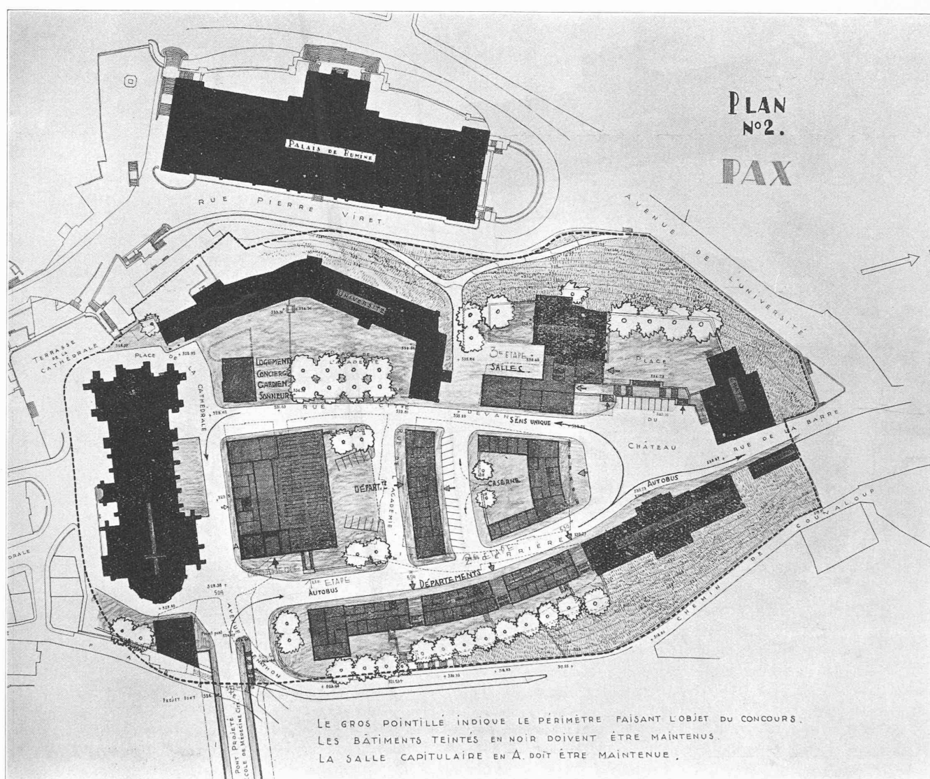
Plan général. — 1 : 2000.
