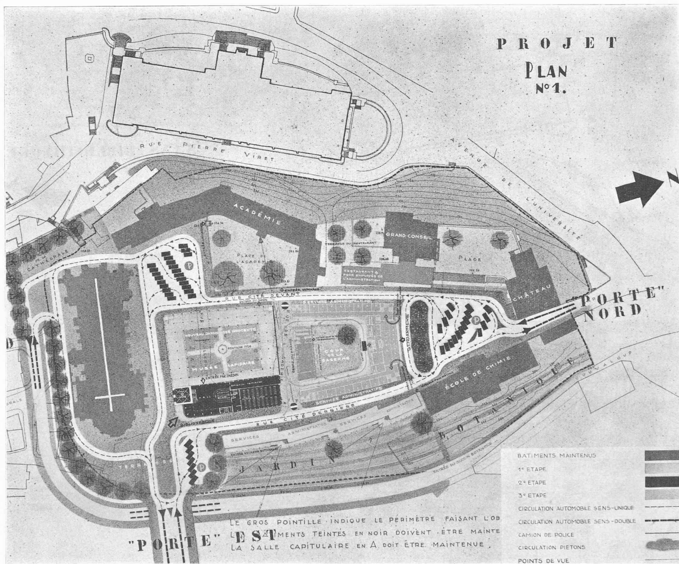
Plan général. — 1 : 2000.
