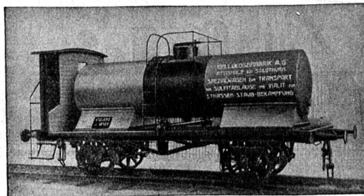
Wagon-Citerne.
