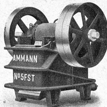
Nouveau concasseur en acier, paliers à rouleaux.
