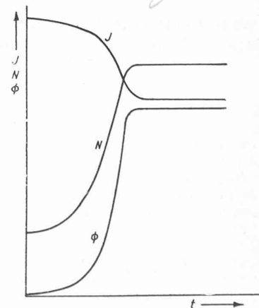
Fig. 12. — Variation de l'intensité de courant, du flux lumineux et du débit électrique, pendant la période d'amorçage de la lampe.
