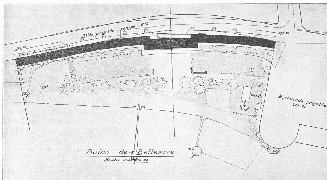
Plan de situation. — 1 : 2000.
