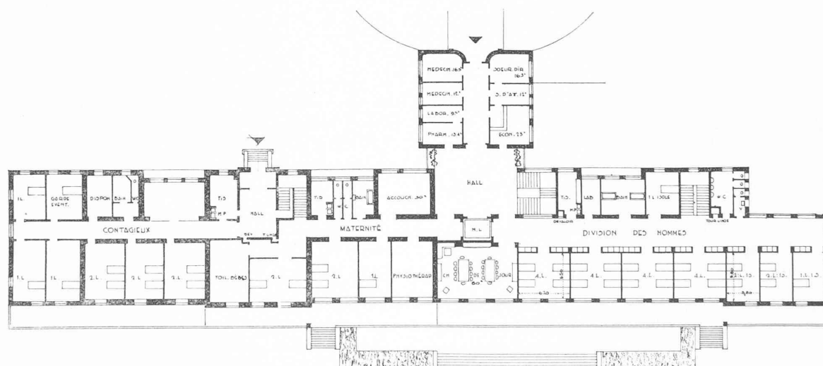
Plan du rez-de-chaussée. — 1 : 600.
