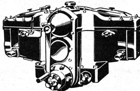
MAG-VICTOR-DIESEL 12 HP
