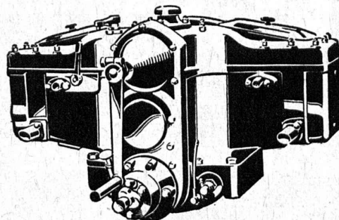
MOTEUR DIESEL MAG-VICTOR 12 HP
