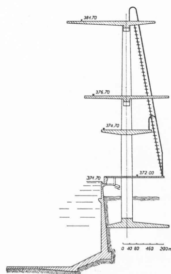
Fig. 4. — Plongeoir olympique à Baden (Suisse).
