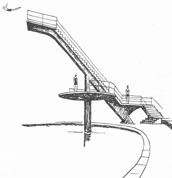
Fig. 2. — Plongeoir à Scarborough (Angleterre). Architecte : Paton-Watson.
