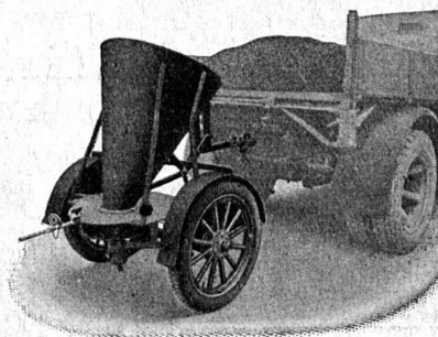
Sableuse derrière camion.
