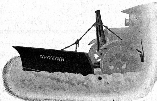
Chasse-neige à lame.
