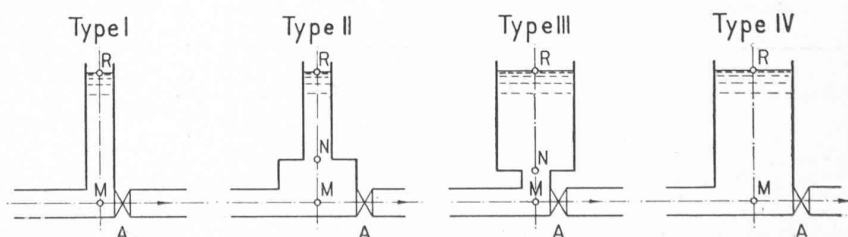
Fig. 5. — Comparaison de divers types de chambres d'équilibre, à l'égard du coup de bélier d'onde.
