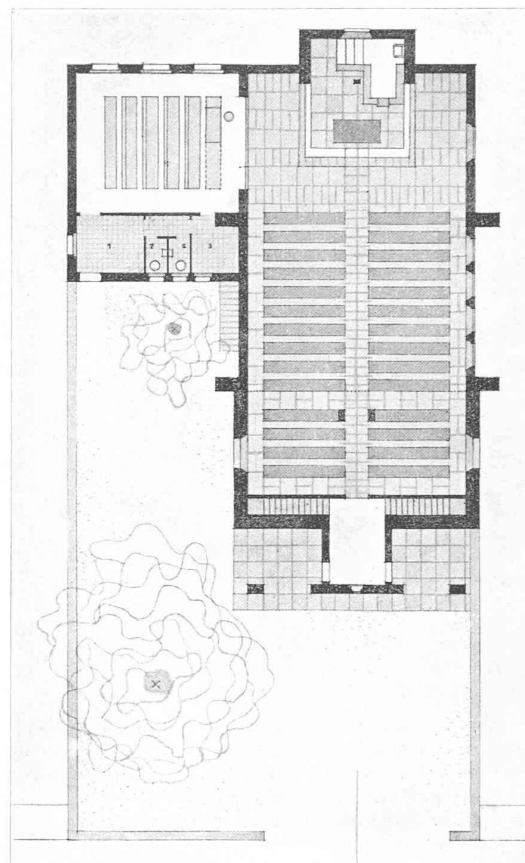
Plan du rez-de-chaussée — 1 : 300.
