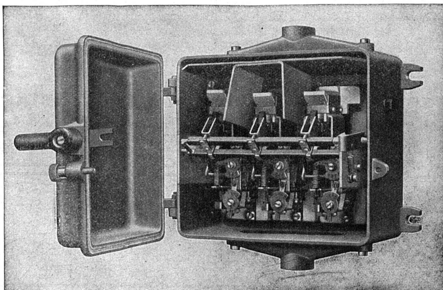
Coffret de manœuvre Type CTFp 7/25
