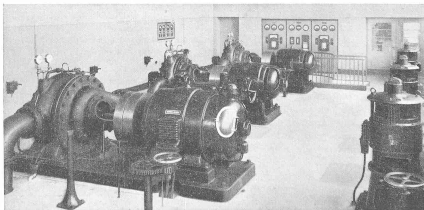
Fig. 5. — Station de pompage à Lutry, des Services industriels de Lausanne, équipée avec 2 télémétrigraphes et 1 conjoncteur-limnimètre Rittmeyer.
