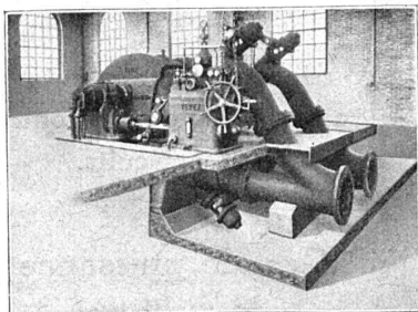
Turbine "Pelton", à 4 injecteurs. (Usine de Sernf-Niederembach.)
