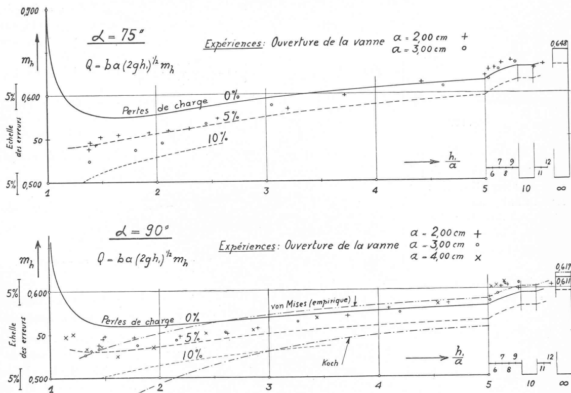
Fig. 19. — \alpha = 75^\circ - 90^\circ . (Voir légende sur figure 17.) Voir, figure 16, perte de charge observées.
