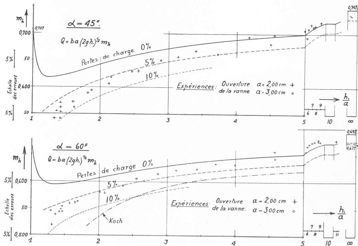
Fig. 18. — \alpha = 45^\circ - 60^\circ . (Voir légende sur figure 17.) Voir, figure 15, pertes de charge observées.
