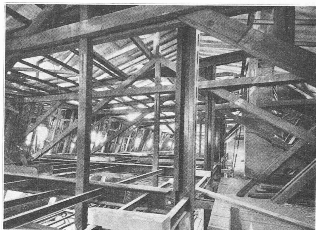
Fig. 9. — Vue du 5 e étage avant l'enlèvement des fermes en bois. Par comparaison avec la figure 5 on se rend compte de la place gagnée par l'adoption de la charpente métallique.
