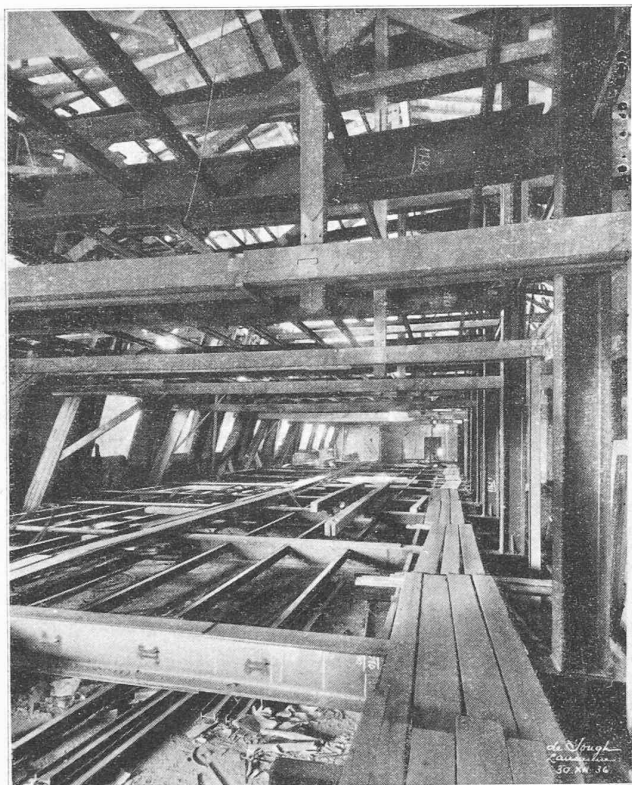
Fig. 4. — Vue du 4 me étage avant l'enlèvement des fermes en bois. Immédiatement au-dessus de l'entrait des fermes en bois apparaissent les sommiers du 5 me étage, dont on distingue les articulations qui les relient aux béquilles.
