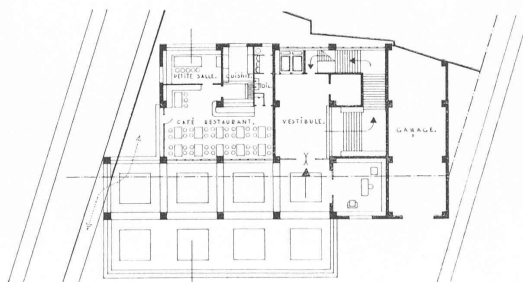
Plan du rez-de-chaussée. 4 : 600.
