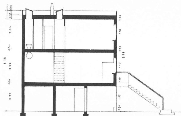
Coupe
