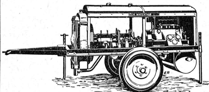
Moto-compresseur "S. L. M. - Winterthur" pour entrepreneurs.
