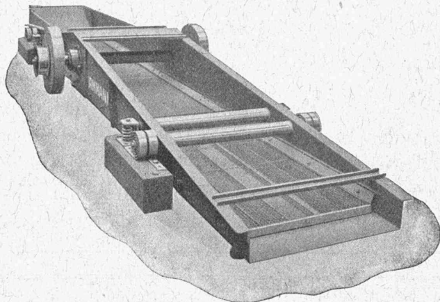
Tamis à oscillations libres assure un tamisage parfait du sable et du gravier
