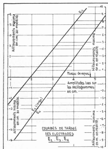
Fig. 28. Courbe de tarage des électrodes, E_2 , E_3 et E_4 .
