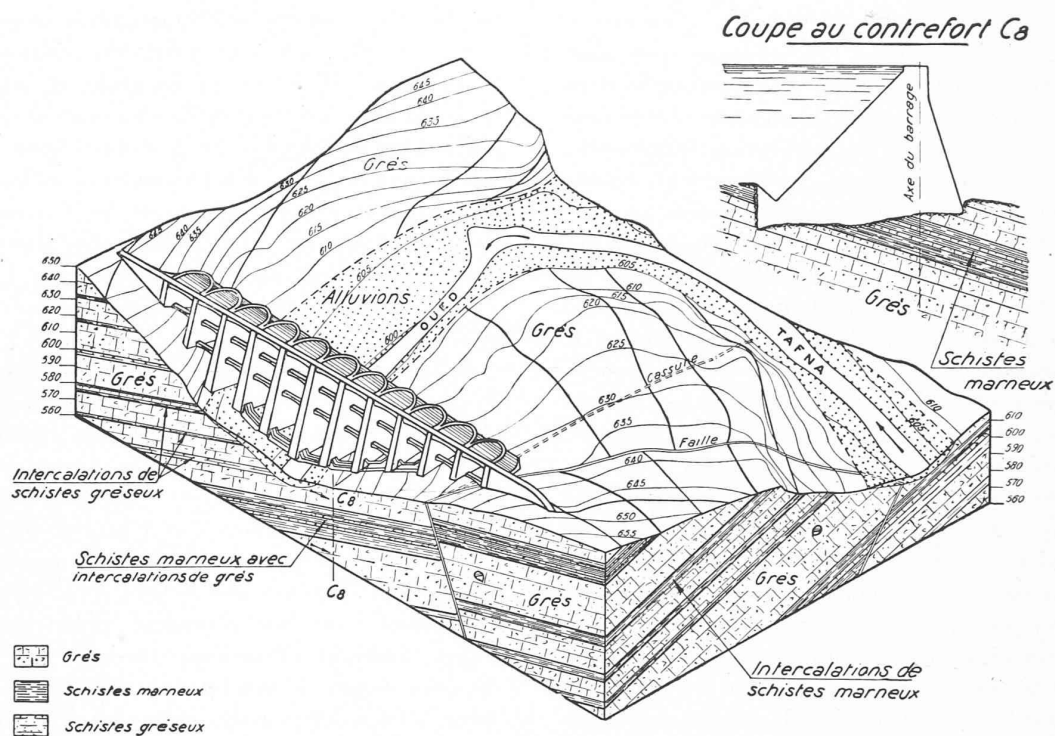
Fig. 1. — Stéréogramme géologique du barrage des Beni-Bahdel près Tlemcen, Algérie. (Dessin d'Alf. Falconnier, géologue). — Les alternances de grès et de schistes plongent à la fois vers l'aval et vers la rive droite. Prédominance des grès sur la rive droite, failles sur la rive gauche. Faible épaisseur d'alluvions sous la Tafna.
