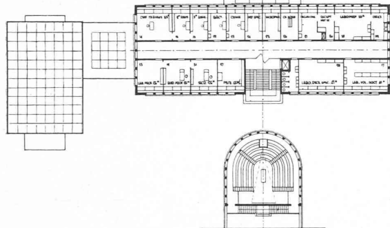
PLAN DU PREMIER ETAGE A: SERVICES DE L'ENSEIGNEMENT
