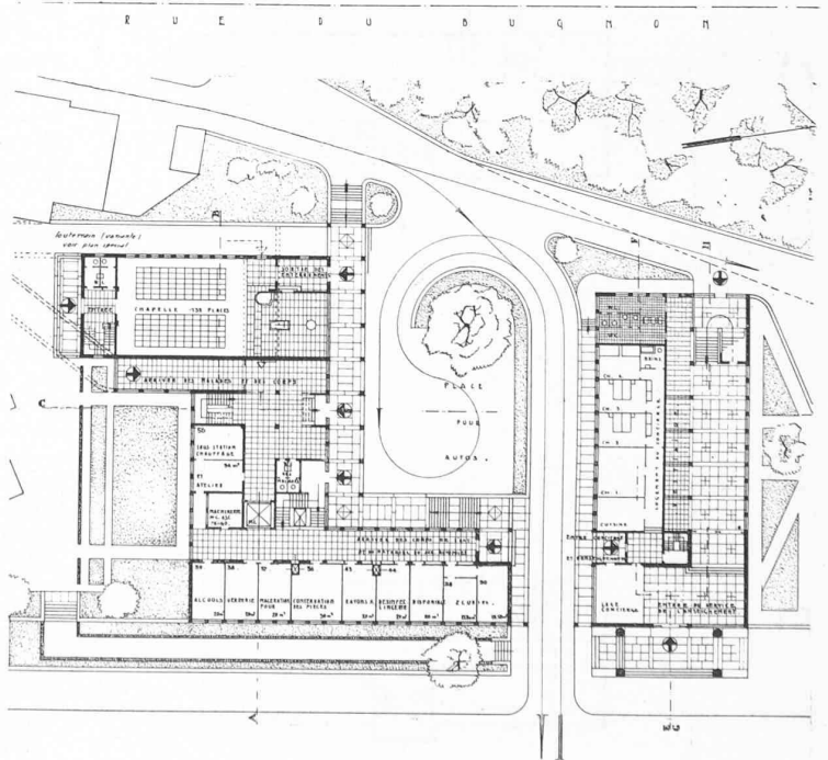
Rez-de-chaussée inférieur et supérieur. — 1 : 800
