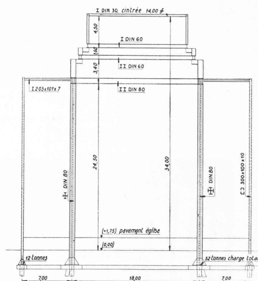
Fig. 5. — Coupe transversale.
