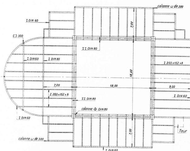
Fig. 3. — Plancher au niveau +23,50.
