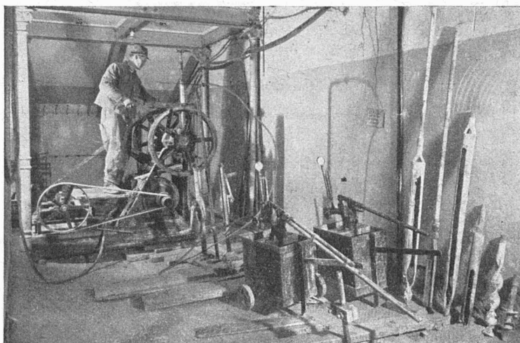
TONHALLE ZURICH Consolidation des fondations avec des injections de ciment et des injections chimiques.
